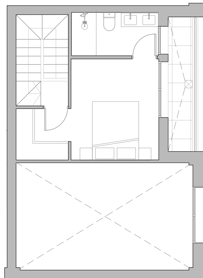
PLANTA PRIMERA
